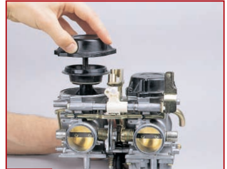
7. Unterdruckkolben ausbauen und Membrane prüfen
