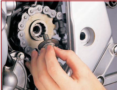
6. Kettenritzel erneuern
