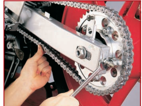
8. Kettenspannung einstellen
